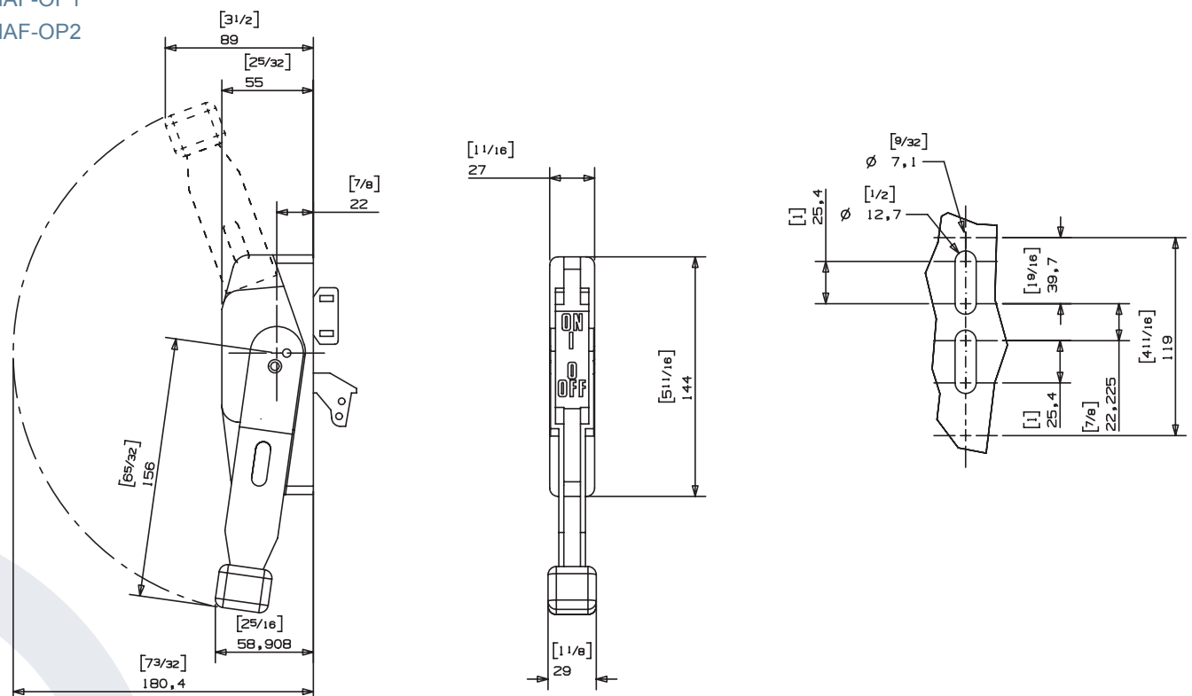
HAF-OP1
